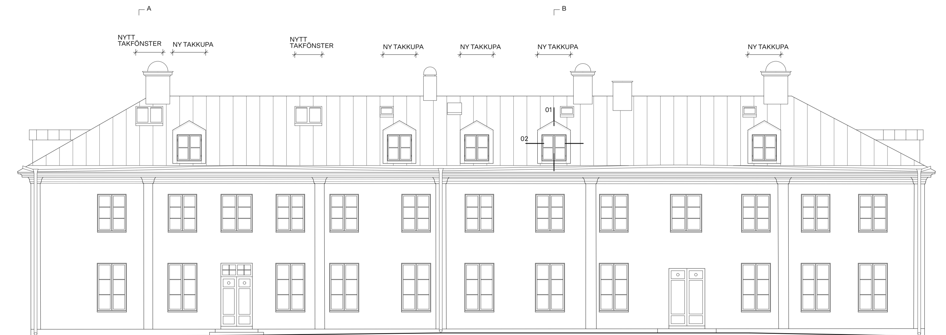
FASAD MOT NORDÖST, GÅRDSFASAD
