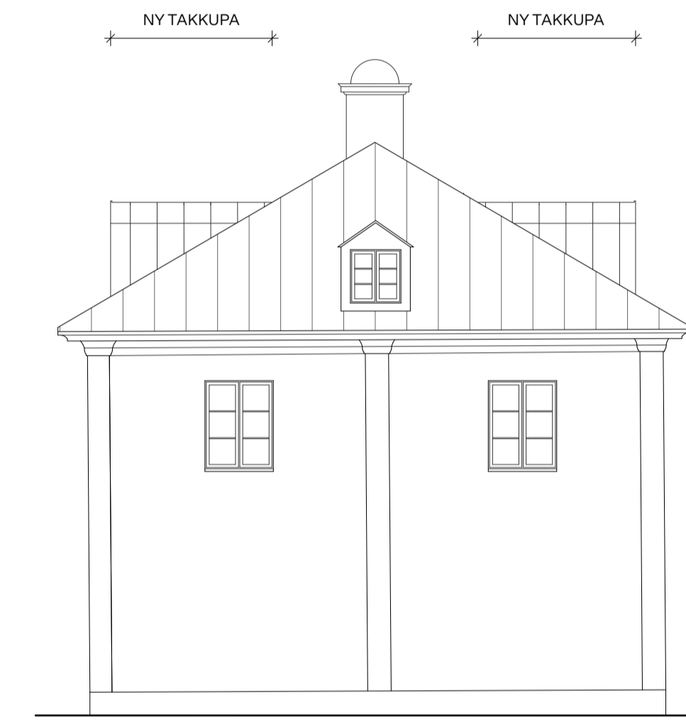
FASAD MOT NORDVÄST
