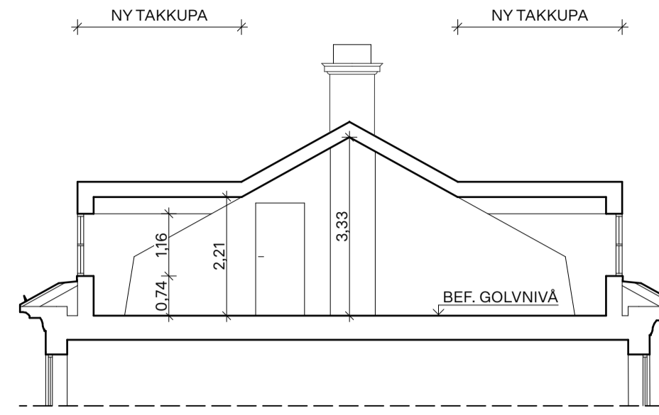
SEKTION B-B
