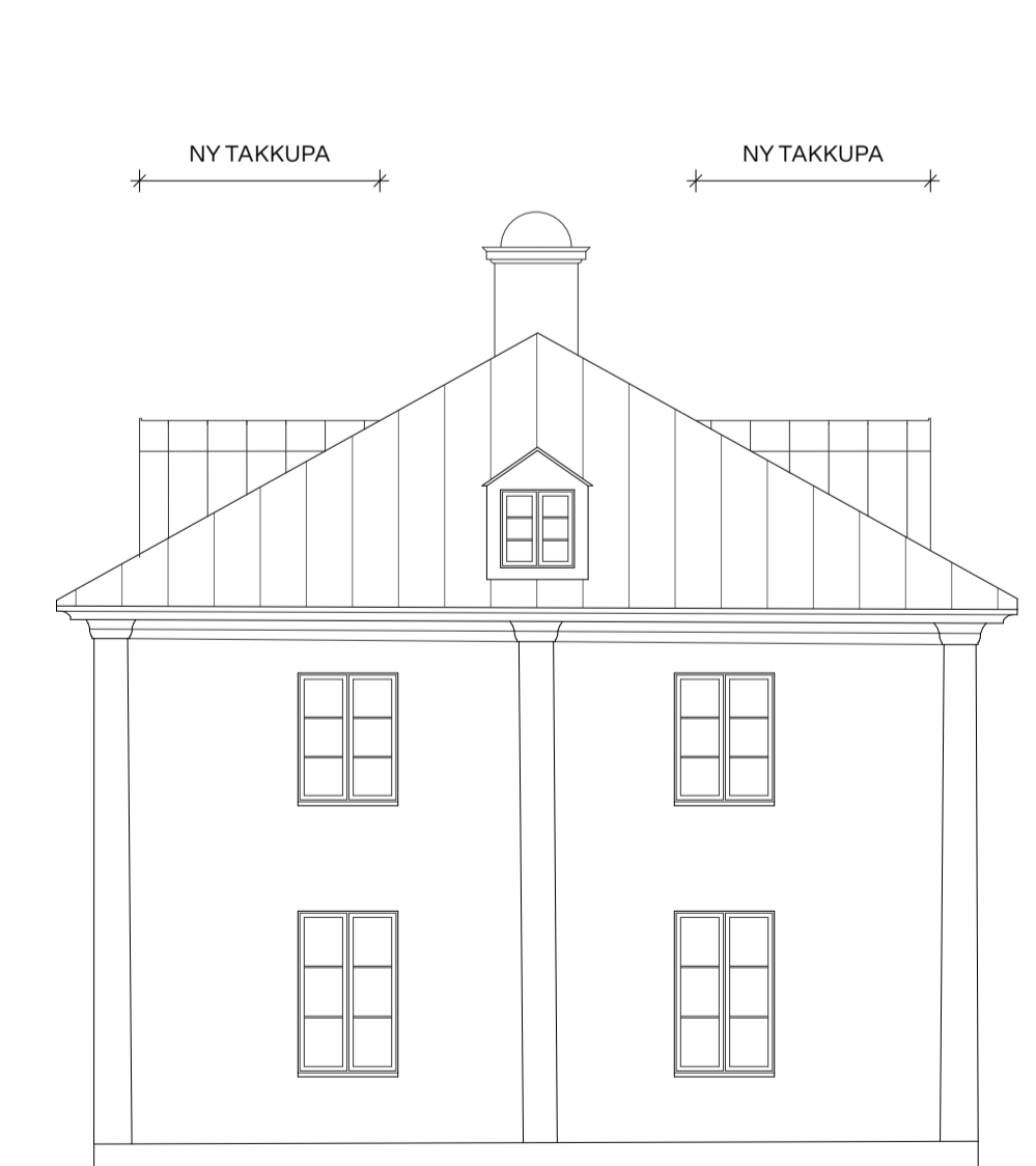
FASAD MOT SYDÖST
