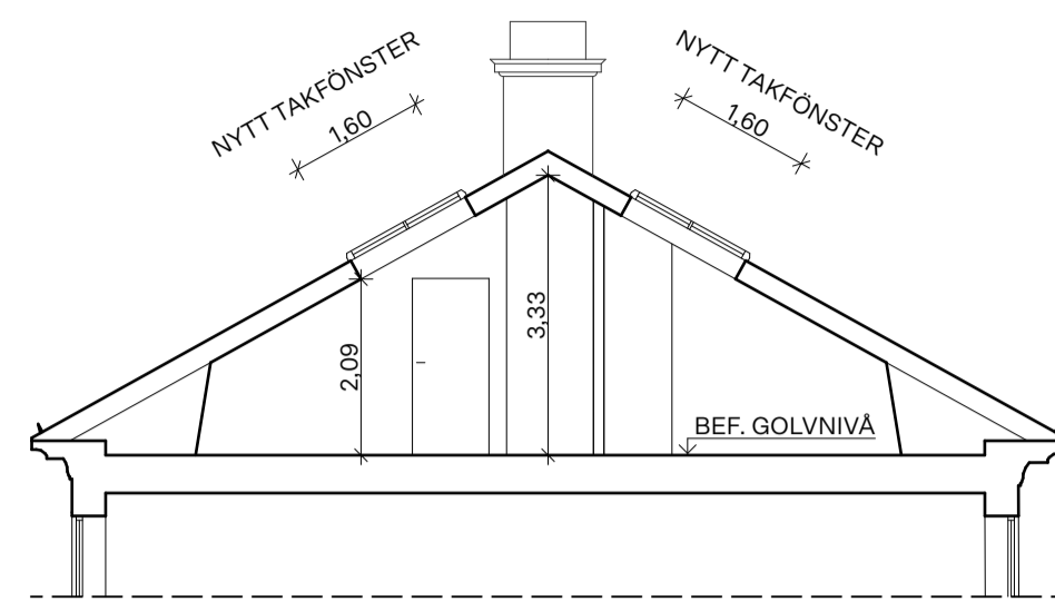
SEKTION A-A
