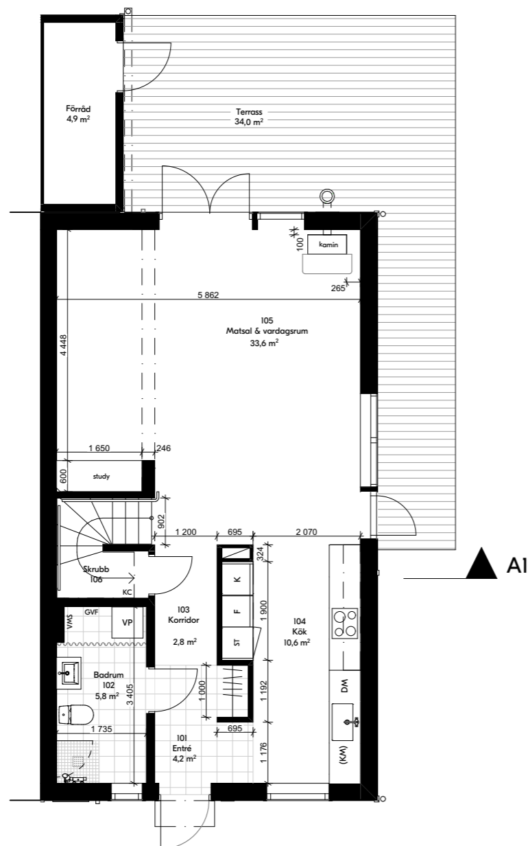
Entréplan
