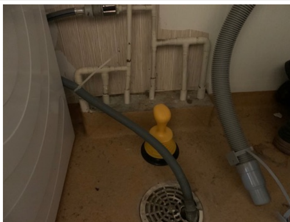
Trycksatta rörgenomföringar i golv
