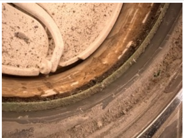
Tätskikt synligt under klämring i golvbrunn
