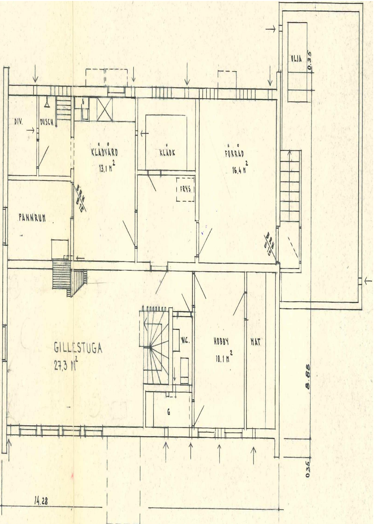
KÄLLARPLAN
